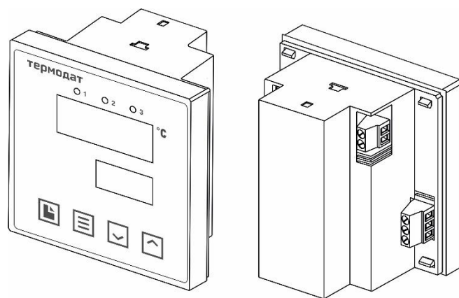
Рисунок 2 – Внешний вид прибора Термодат-10К7-М
