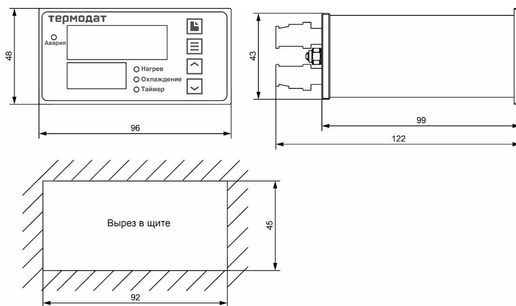
Рисунок 29 – Габаритные размеры прибора Термодат-10К7-Н
