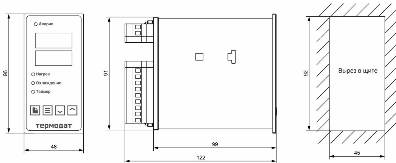
Рисунок 28 – Габаритные размеры прибора Термодат-10К7-В
