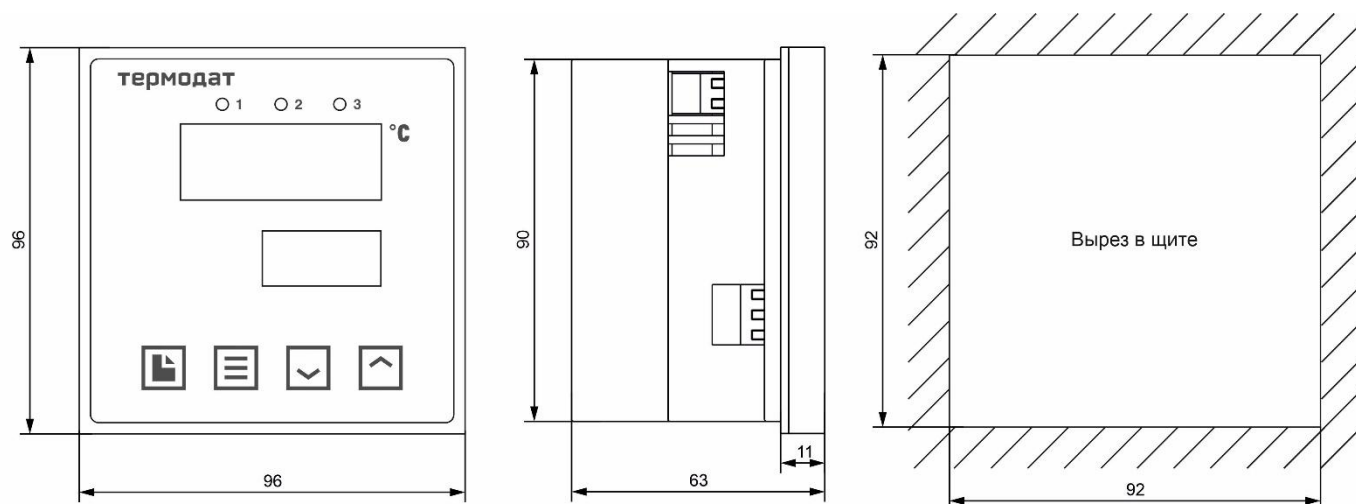
Рисунок 26 – Габаритные размеры прибора Термодат-10К7-М
