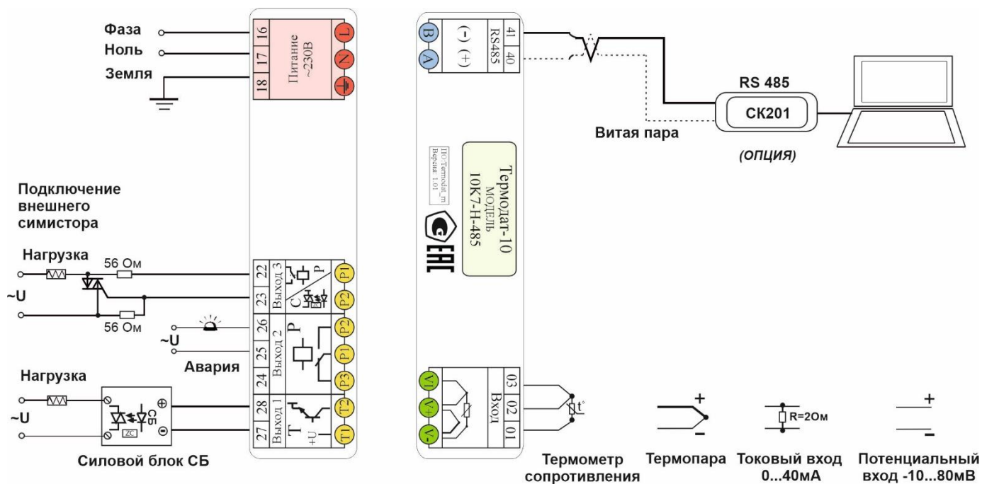
Рисунок 22 – Схема подключения прибора Термодат-10К7-Н-485
