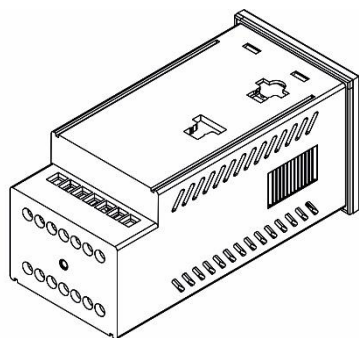
Рисунок 5 – Внешний вид прибора Термодат-10К7-К
