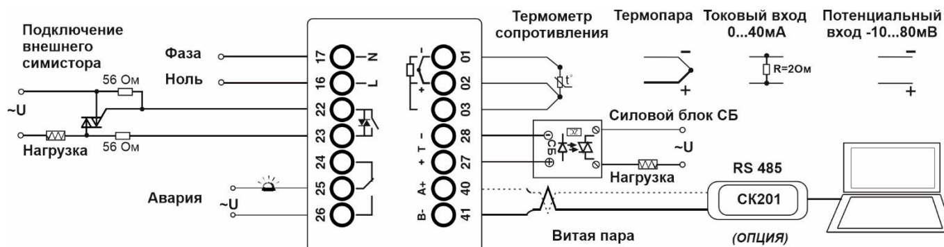
Рисунок 23 – Схема подключения прибора Термодат-10К7-К-485
