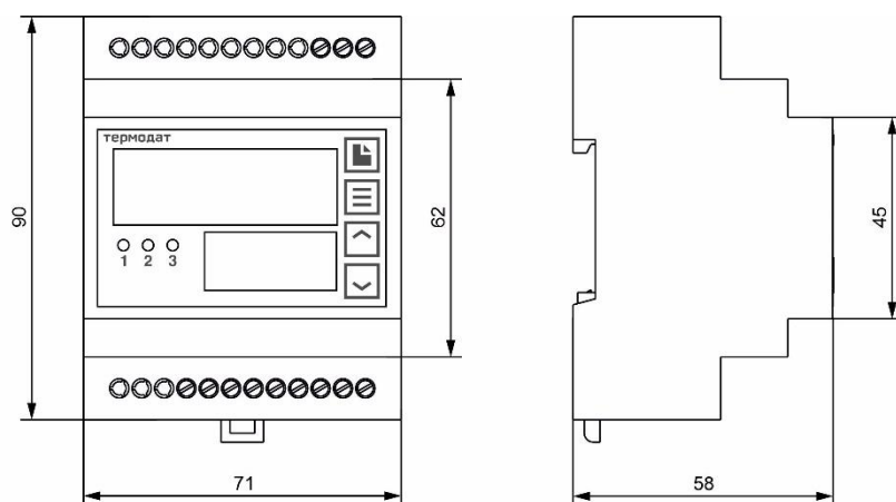
Рисунок 29 – Габаритные размеры прибора Термодат-10К7-Н
