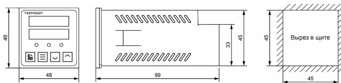
Рисунок 27 – Габаритные размеры прибора Термодат-10К7-К
