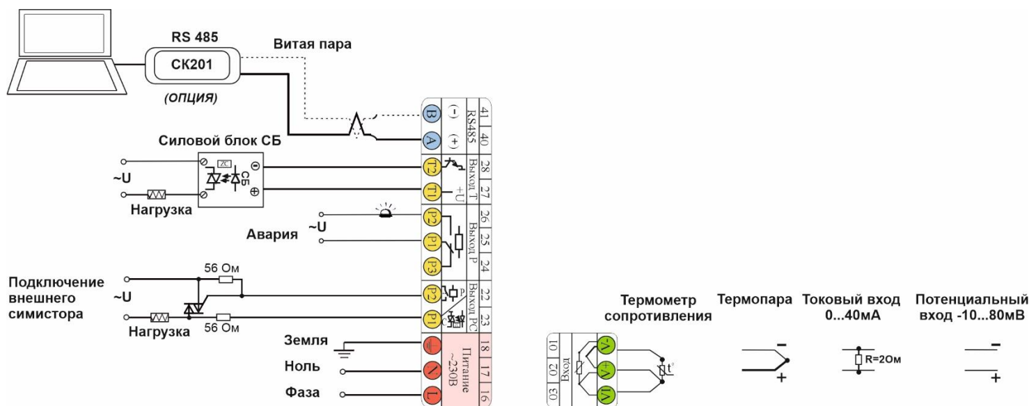
Рисунок 24 – Схема подключения прибора Термодат-10K7-P4-485
