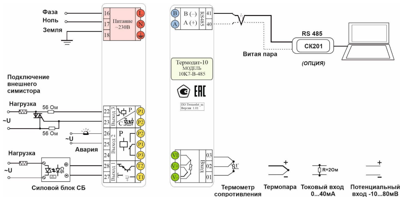
Рисунок 21 – Схема подключения прибора Термодат-10К7-В-485
