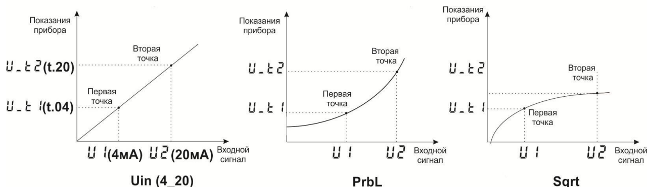
Рисунок 10 – Графики зависимости показаний прибора от входного сигнала при использовании входа типа U.in , PrbL , SqrL и датчика 4...20
