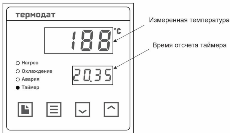
Рисунок 11 - Внешний вид прибора с включенным таймером
