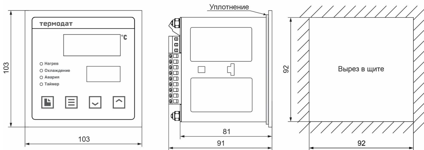
Рисунок 20 – Габаритные размеры прибора Термодат-12К6-А...
