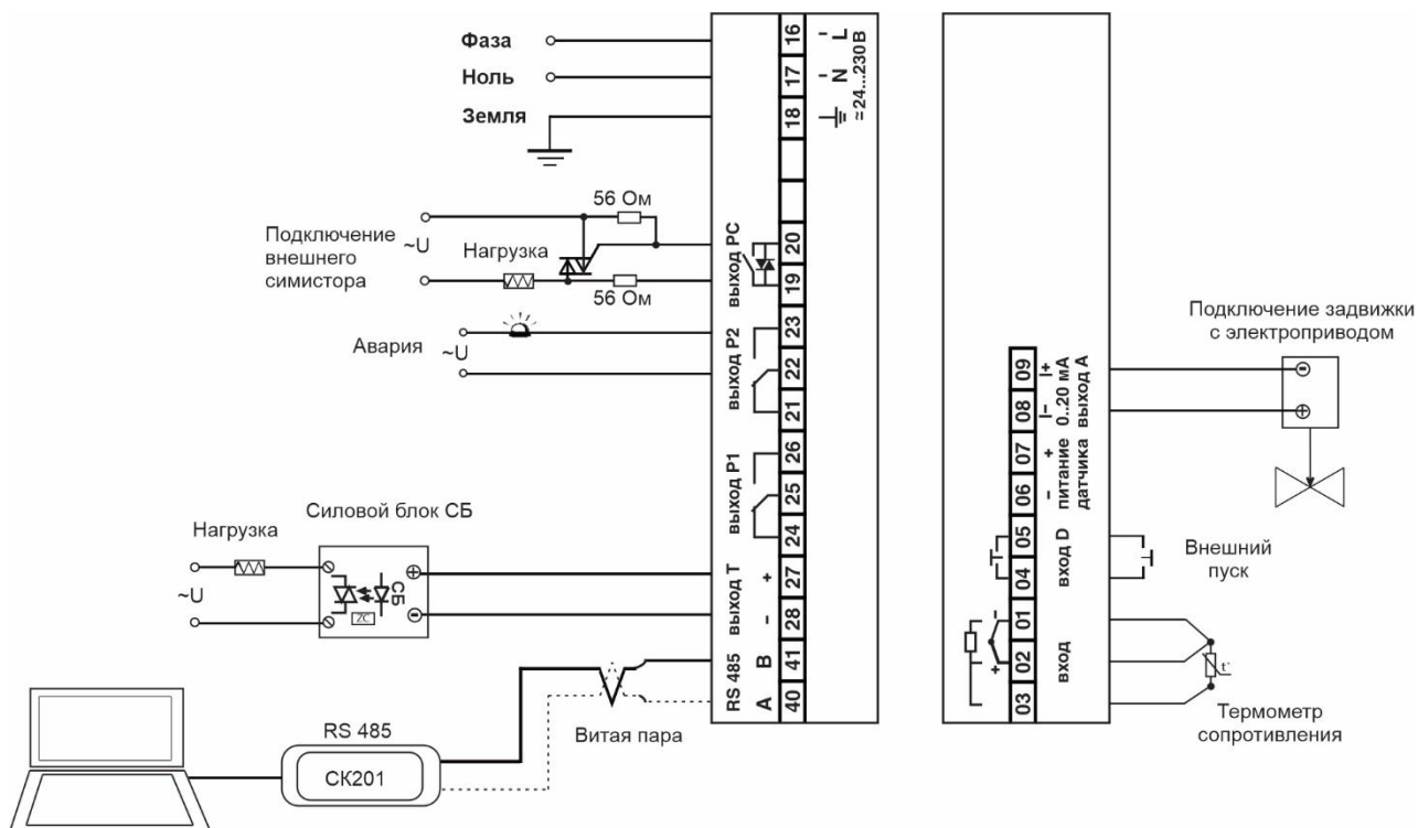
Рисунок 11 – Схема подключения прибора
