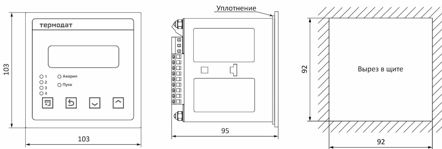
Рисунок 14 – Габаритные размеры прибора Термодат-14Е5-А7-4М
