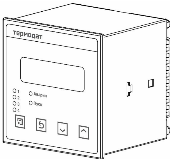
Рисунок 1 – Внешний вид прибора Термодат-14Е5-А...
