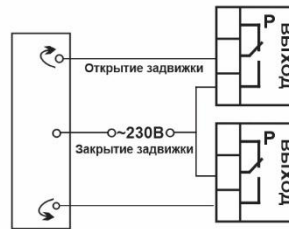
Подключение электродвигателя
