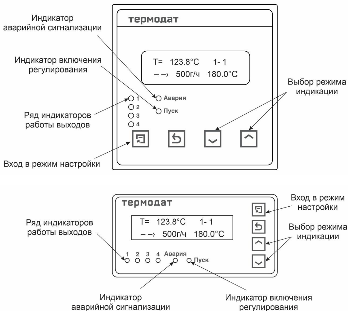
Рисунок 3 – Описание индикаторов и кнопок управления прибора
