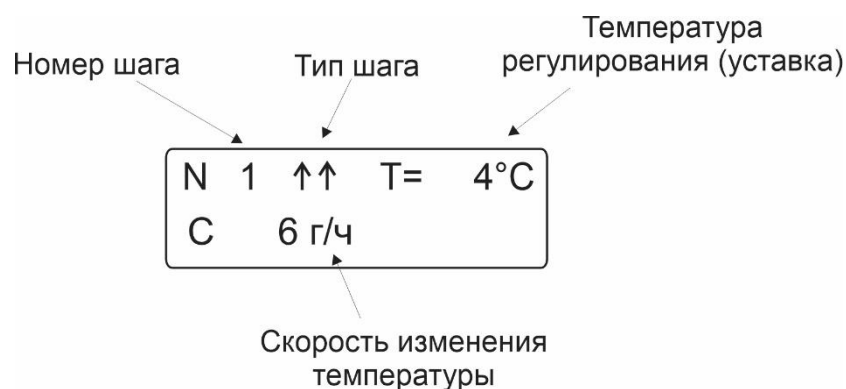
Рисунок 5 – Отображение редактора программ на дисплее прибора
