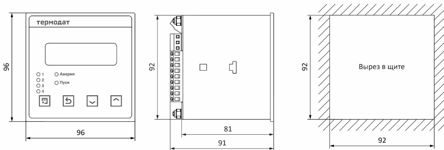
Рисунок 13 – Габаритные размеры прибора Термодат-14Е5-А...
