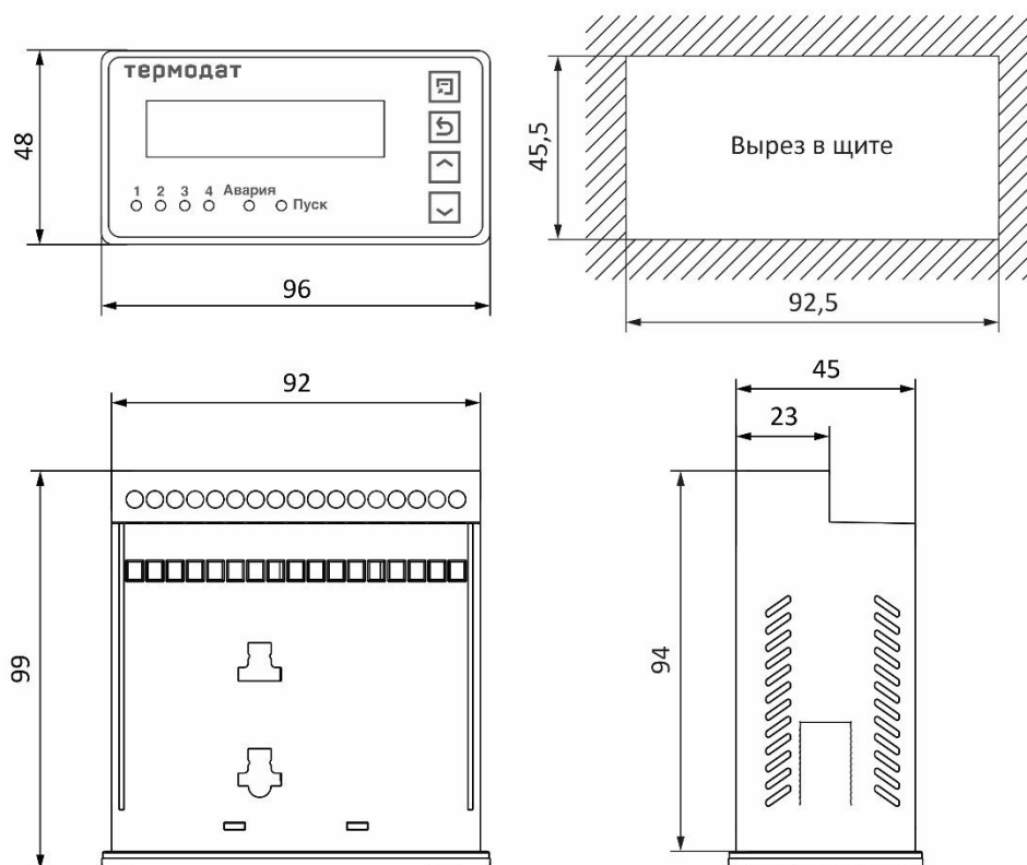
Рисунок 12 – Габаритные размеры прибора Термодат-14Е5-Н...
