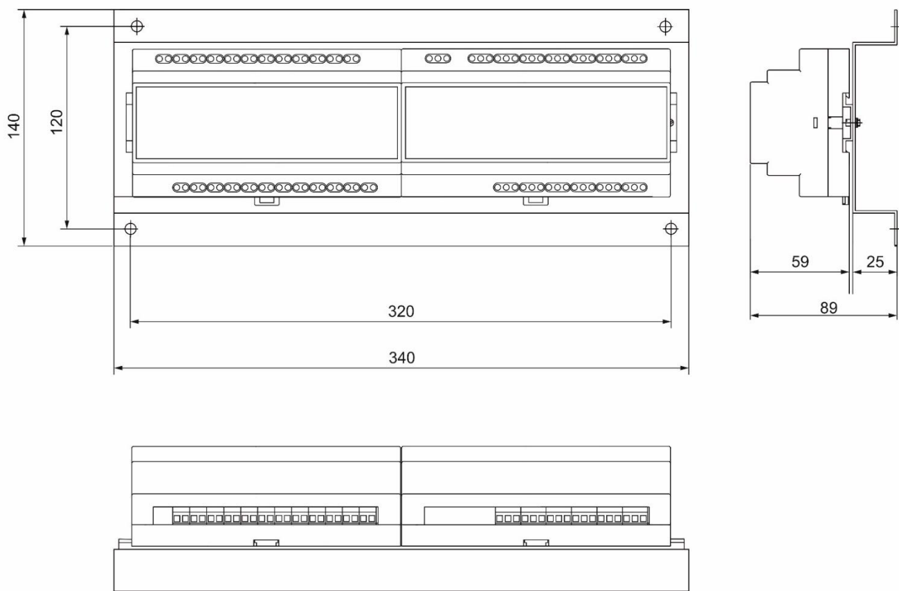
Рисунок 15 – Габаритные размеры блока измерения и блока выходов РВ/8(12)УВ/8(12)Р(Т,С)/(8(12)Р)
