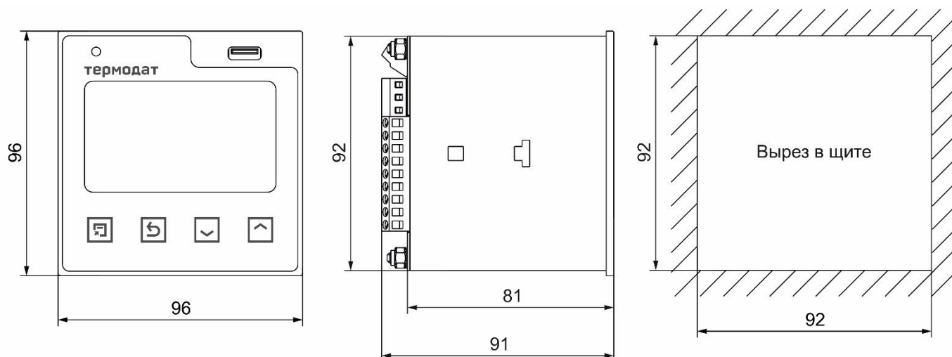
Рисунок 13 – Габаритные размеры основного блока прибора Термодат-25Е6/...../F
