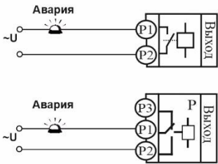
Подключение аварийной сигнализации
