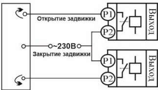
Подключение электрозадвижки
