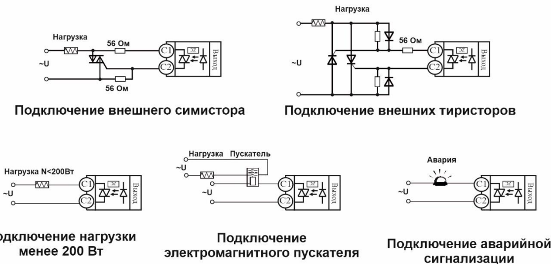
Рисунок 10 – Схемы подключения симисторного выхода
