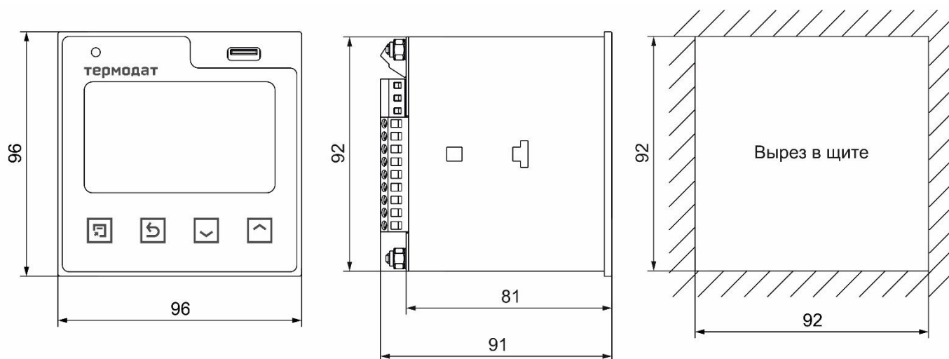
Рисунок 7 – Габаритные размеры прибора Термодат-25М6/...../F
