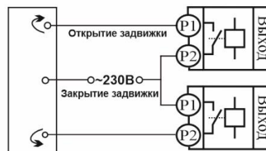
Подключение электрозадвижки
