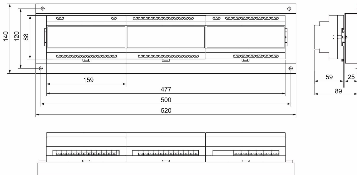
Рисунок 11 – Габаритные размеры блока измерения, блока выходов и блока аналоговых выходов РВ/12УВ/12Р/12Р-12А
