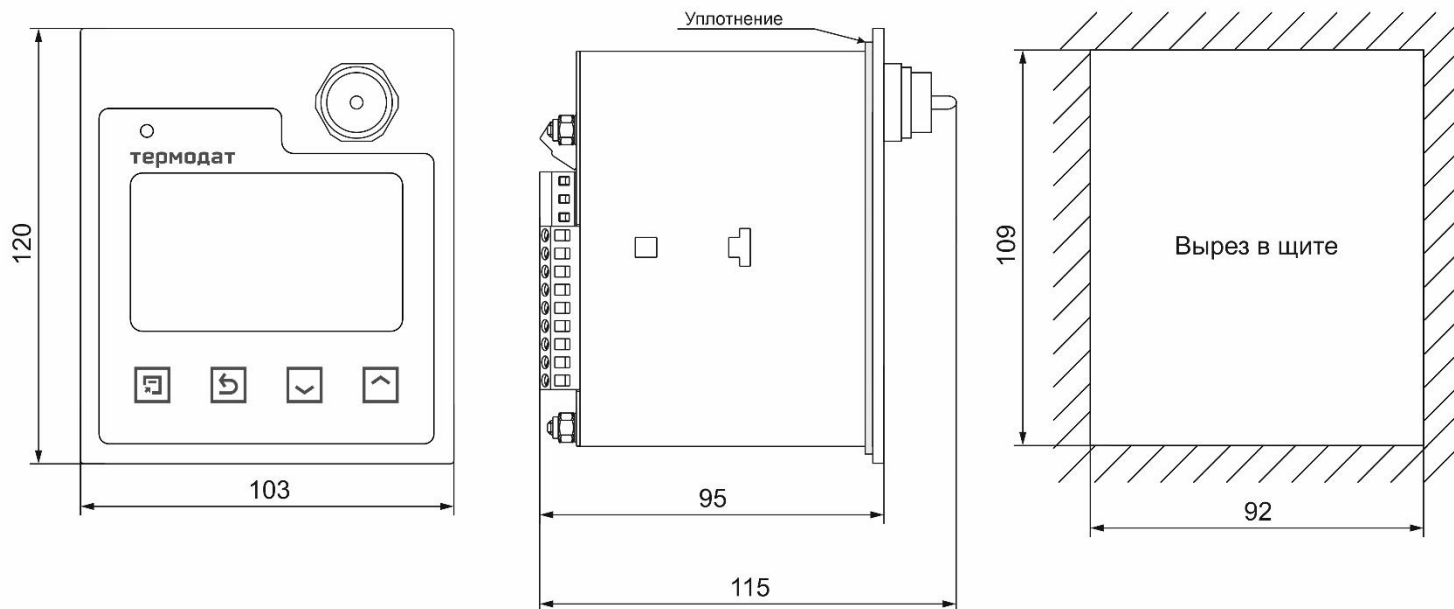
Рисунок 7 – Габаритные размеры прибора Термодат-25М6/...../F
