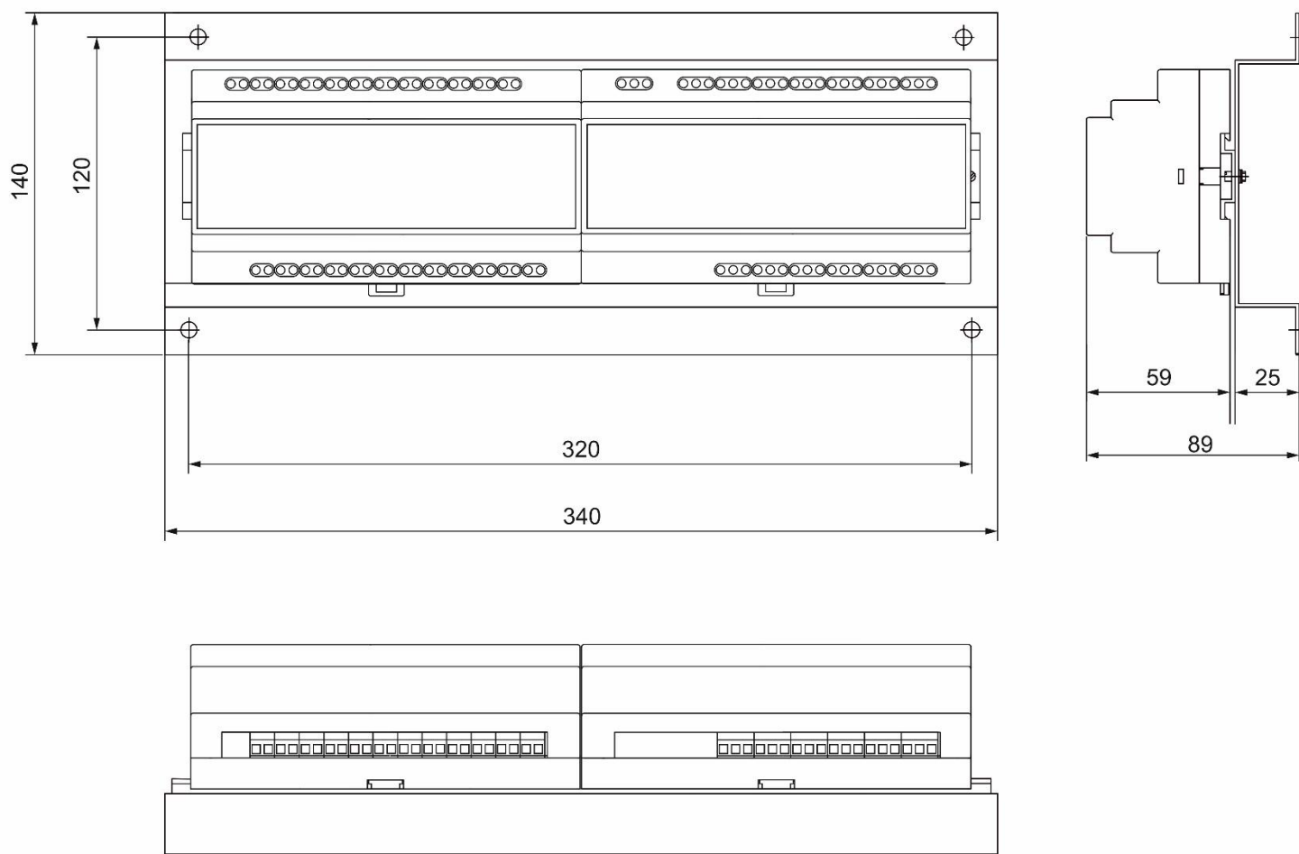
Рисунок 9 – Габаритные размеры блока измерения RV4/8УВ(12УВ)
