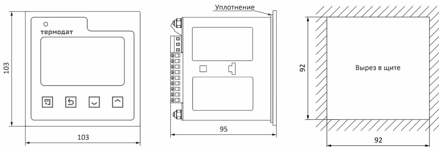
Рисунок 15 – Габаритные размеры прибора Термодат-16Е6-А-(F)-(Eth)
