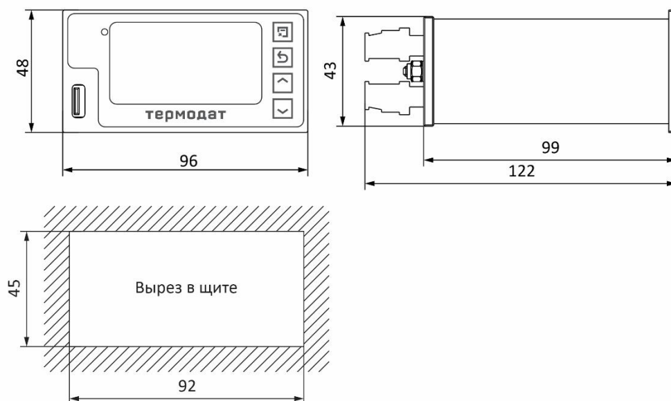
Рисунок 18 – Габаритные размеры прибора Термодат-16Е6-Н-(F)-(Eth)
