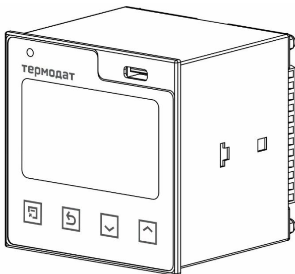
Рисунок 1 – Внешний вид прибора Термодат-16E6-A...
