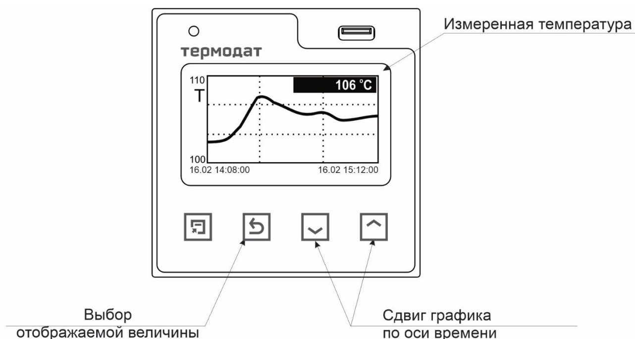
Рисунок 5 - Режим индикации «График»
