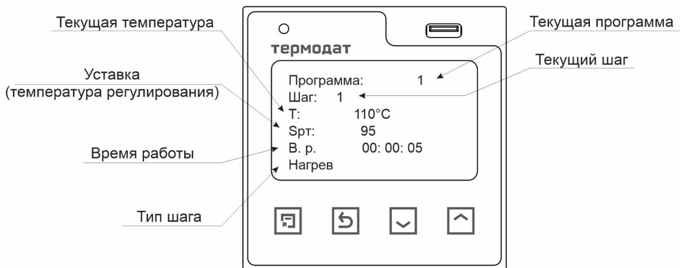
Рисунок 4 - Режим индикации «Текст- состояние программы»
