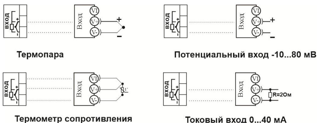
Рисунок 9 – Схемы подключения датчиков
