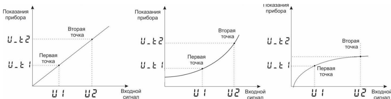
Рисунок 7 – Графики линейной, квадратичной зависимости или зависимости с извлечением квадратного корня для входа
