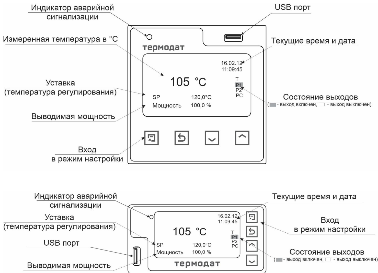
Рисунок 3 - Режим индикации «Текст- значение крупно»
