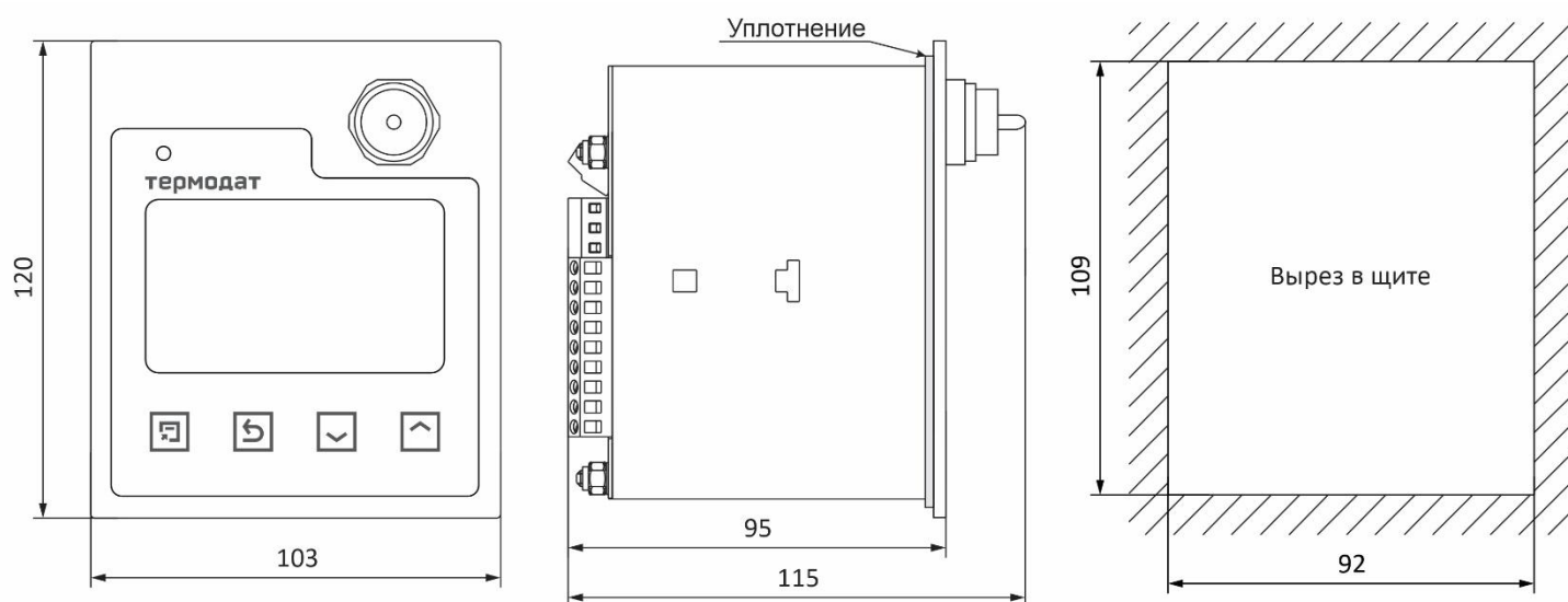
Рисунок 17 – Габаритные размеры прибора Термодат-16Е6-А9-Е
