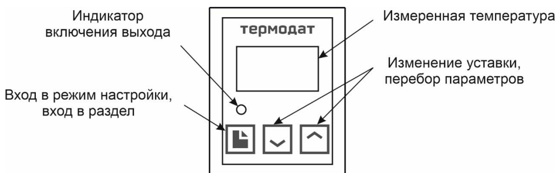
Рисунок 1 – Описание индикаторов и кнопок управления прибором
