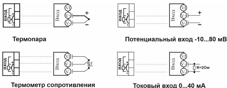
Рисунок 4 – Схема подключения датчиков температуры
