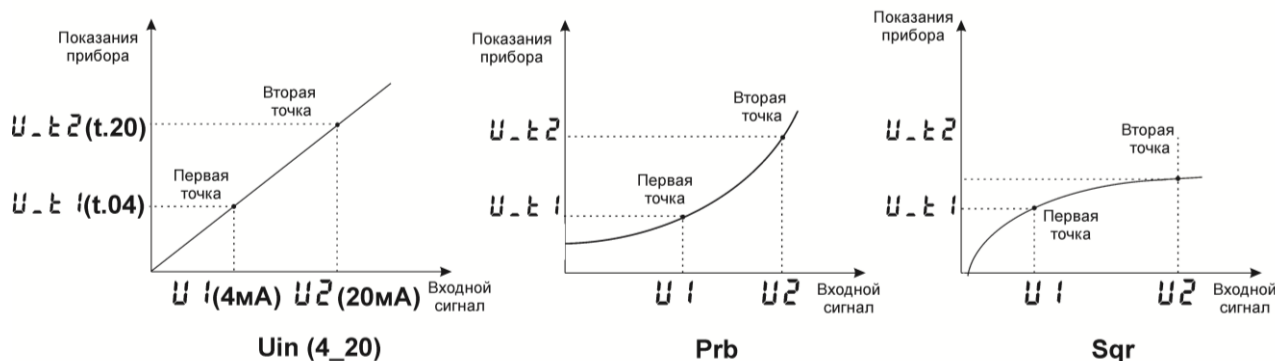
Рисунок 3 – Графики зависимости показаний прибора от входного сигнала при использовании входа типа U.in , Prb , Sqr и датчика 4.20
