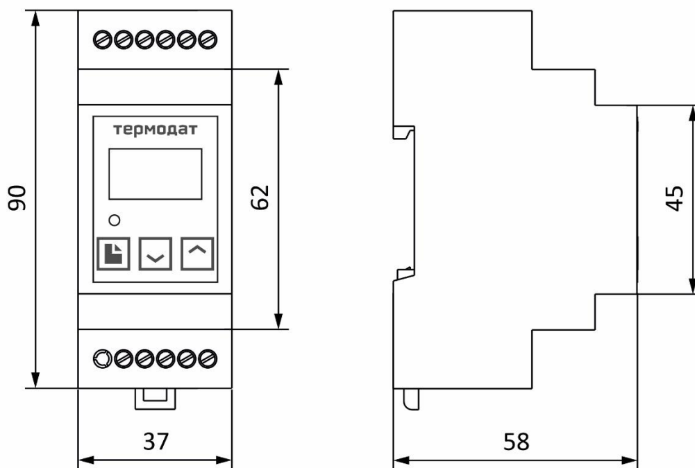
Рисунок 9 – Габаритные размеры прибора
