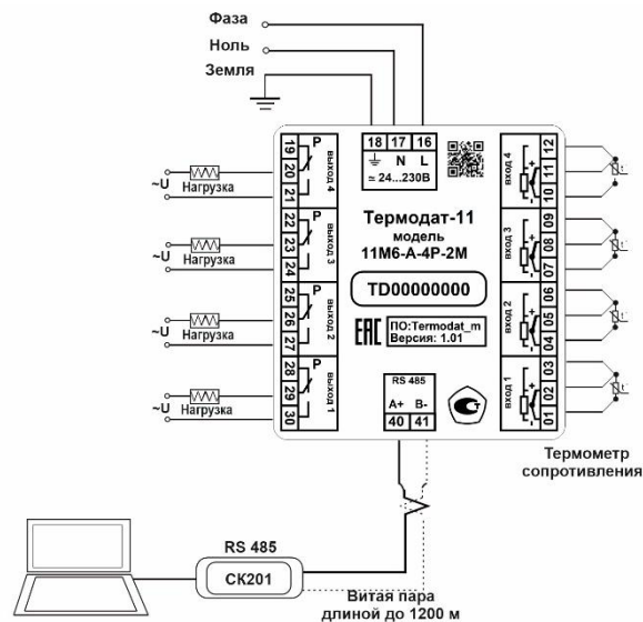
Рисунок 14 - Схема подключения Термодат -11М6-А... для регулирования температуры по четырем каналам
