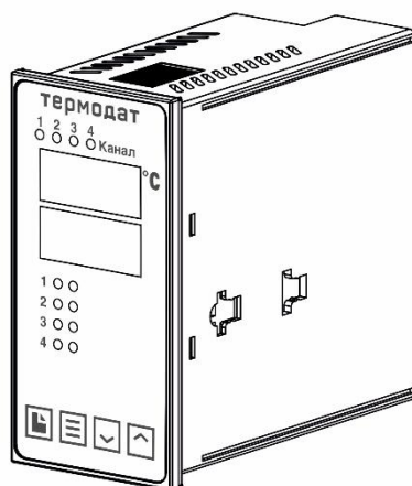
Рисунок 3 – Внешний вид прибора Термодат-11М6-В...
