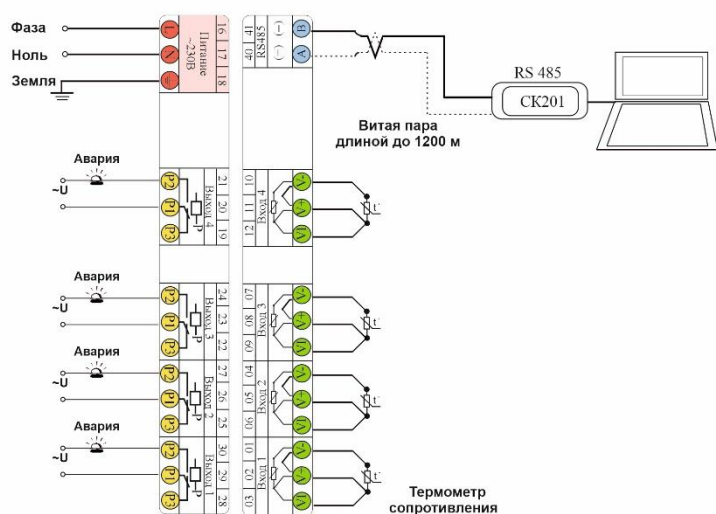
Рисунок 15 - Схема подключения Термодат -11М6-Р6... при использовании прибора как аварийного сигнализатора, напряжение питания 230В
