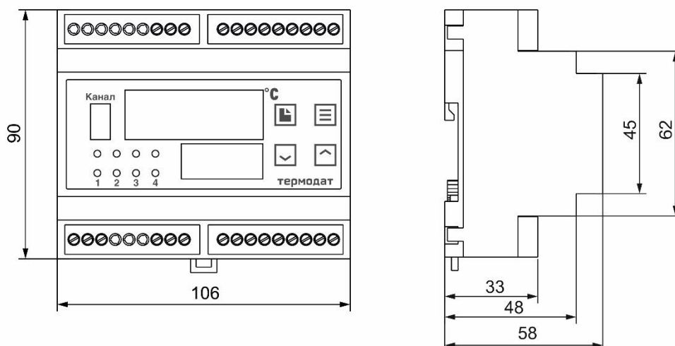
Рисунок 19 – Габаритные размеры прибора 11М6-Р6...
