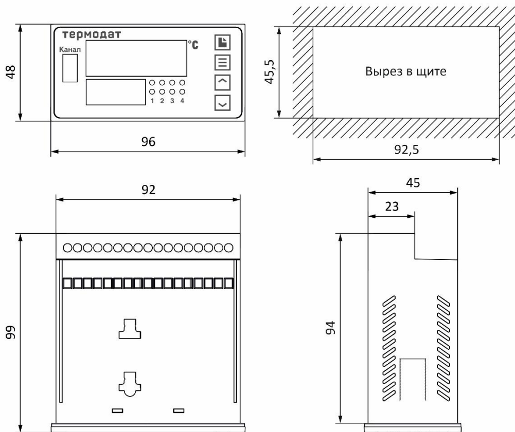
Рисунок 20 – Габаритные размеры прибора 11М6-В...
