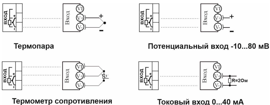
Рисунок 10 – Схема подключения датчиков температуры
