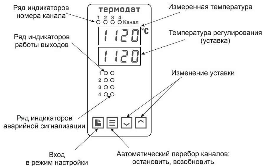
Рисунок 7 – Описание индикаторов и кнопок управления приборов 11М6-В...
