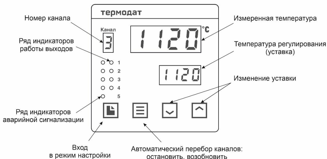
Рисунок 5 – Описание индикаторов и кнопок управления приборов 11М6-А...
