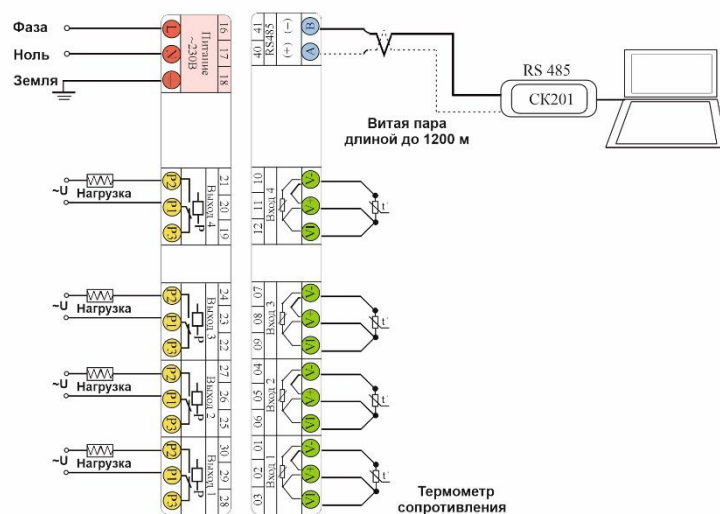
Рисунок 16 - Схема подключения Термодат -11М6-Р6... для регулирования температуры по четырем каналам
