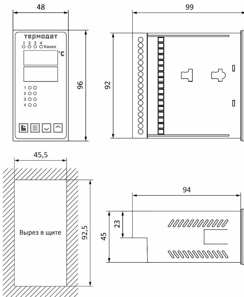
Рисунок 20 – Габаритные размеры прибора 11М6-В...
