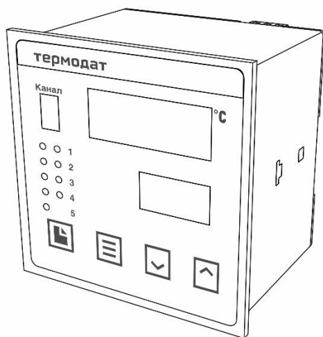
Рисунок 1 – Внешний вид прибора Термодат-11М6-А...
