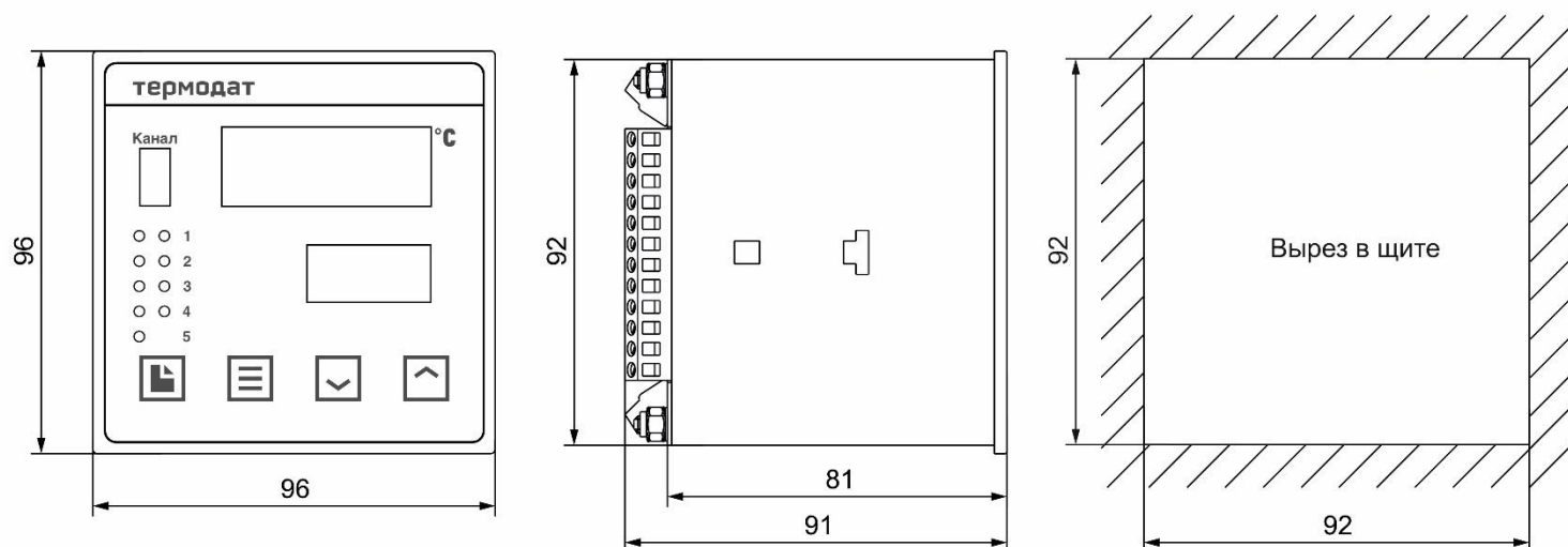
Рисунок 17 – Габаритные размеры прибора 11М6-А...
