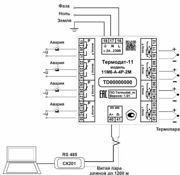
Рисунок 13 - Схема подключения Термодат -11М6-А... при использовании прибора как аварийного сигнализатора, напряжение питания 230В
