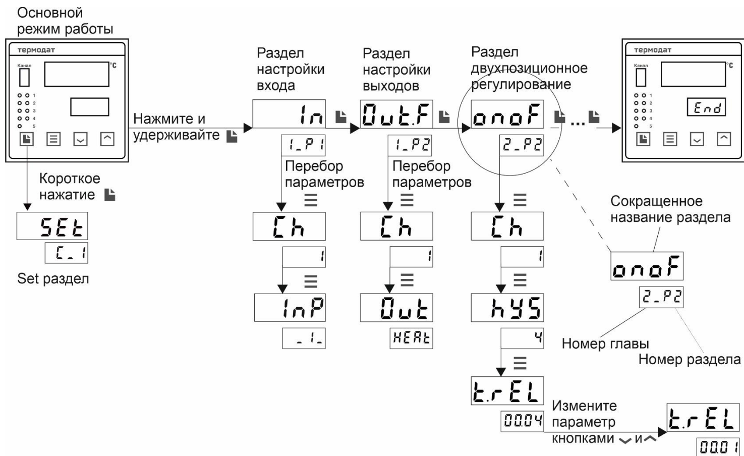
Рисунок 9 – Схема меню настройки прибора 11М6-А...
