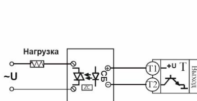
Управление однофазной нагрузкой с помощью блока СБ
