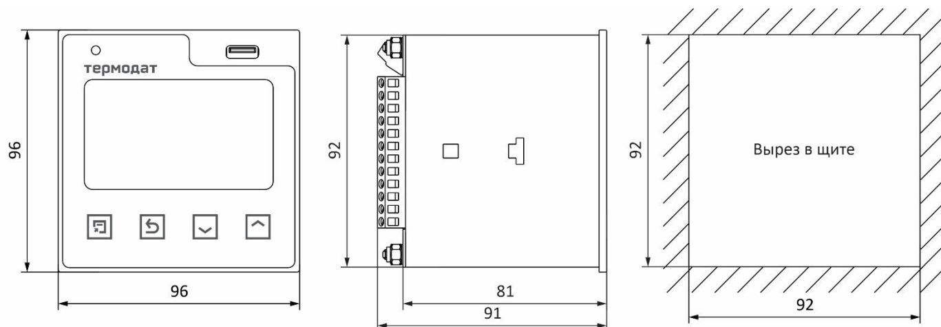
Рисунок 14 – Габаритные размеры прибора Термодат-17Е6/...../(F)
