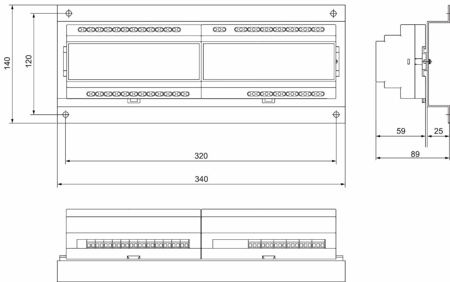
Рисунок 7 – Габаритные размеры блока измерения и блока выходов RV/8(12)УВ/8(12)P/(8(12)P)
